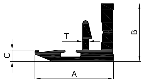
INDUSTRIAL SECTION (VAF)
